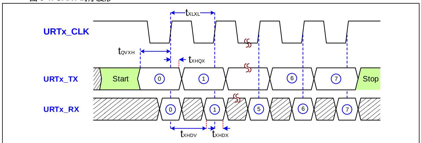
图 8-1. UART 时序波形
