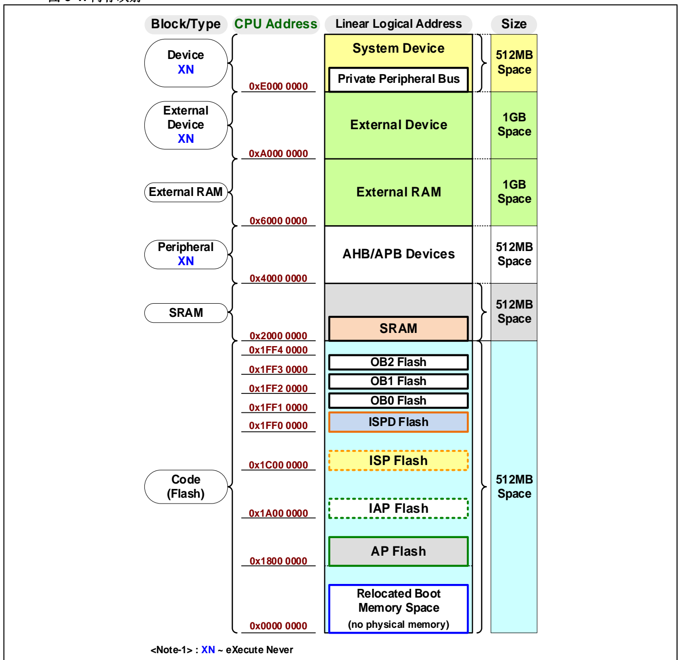
图 5-1. 内存映射
