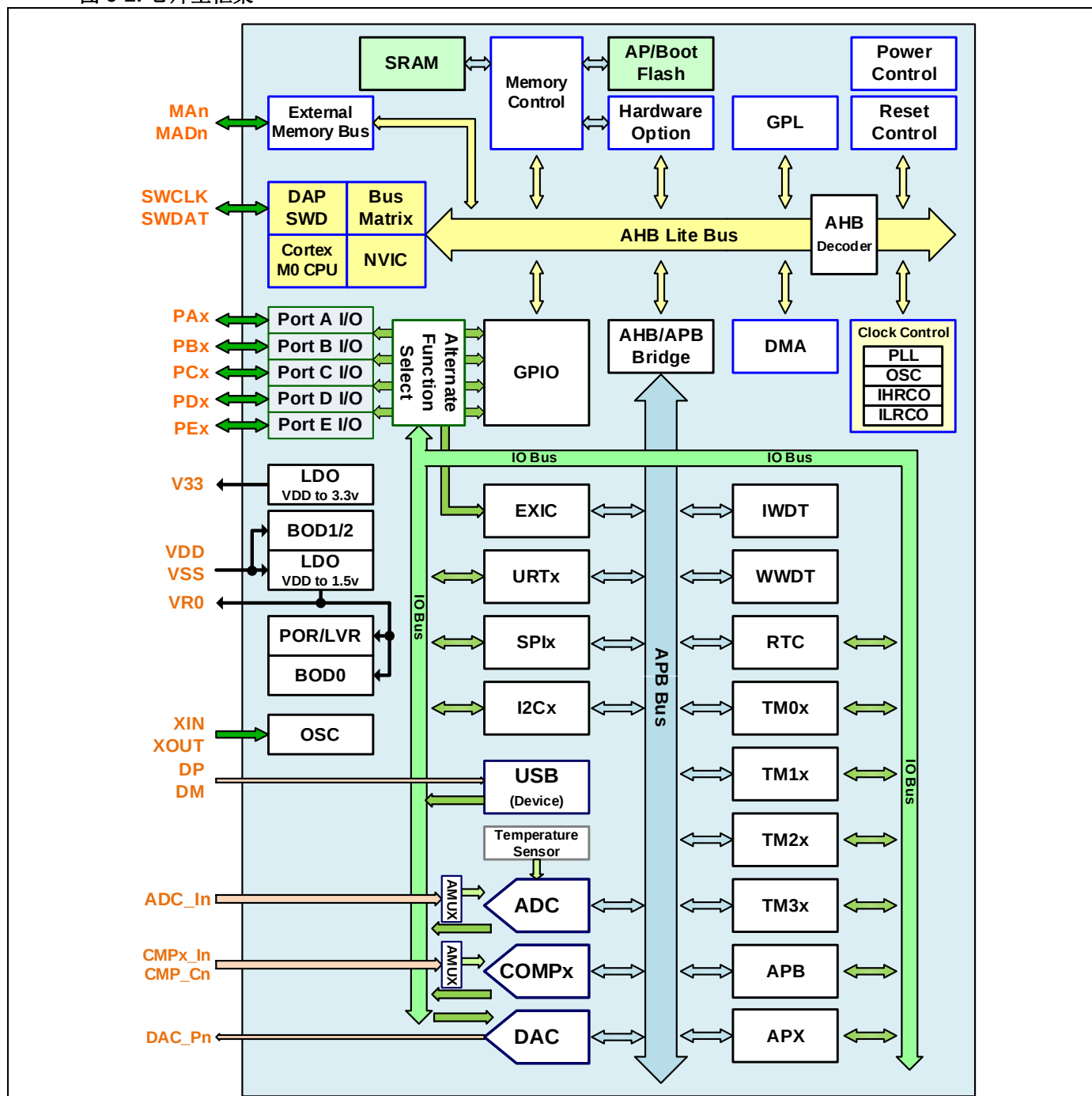
图 3-2. 芯片主框架
