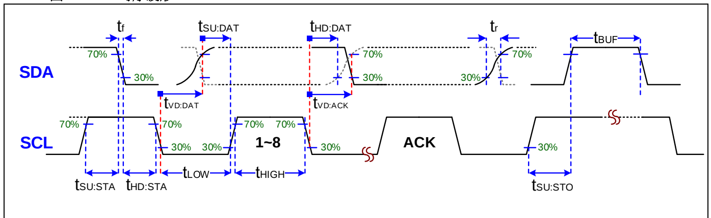
图 8-4. I2C 时序波形
