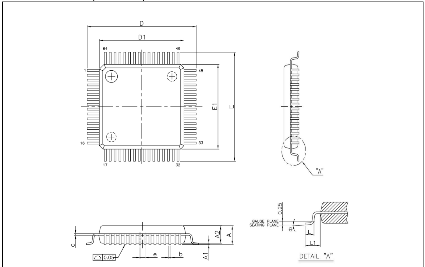
图 9-2. LQFP-64 (7mm X 7mm) ~ AD64
